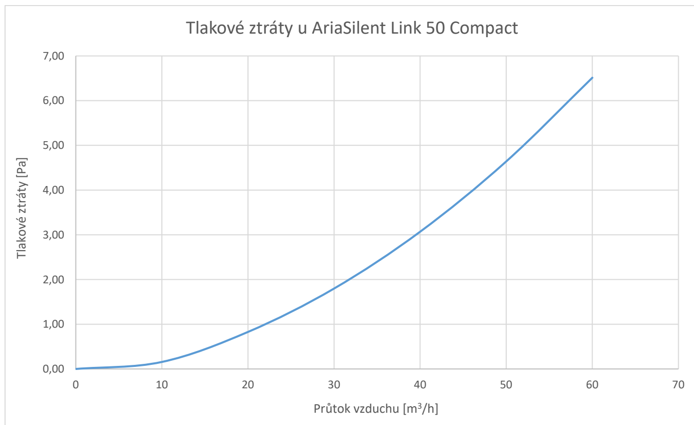
Obrázek: Tlakové ztráty u AriaSilent Link Compact 50
