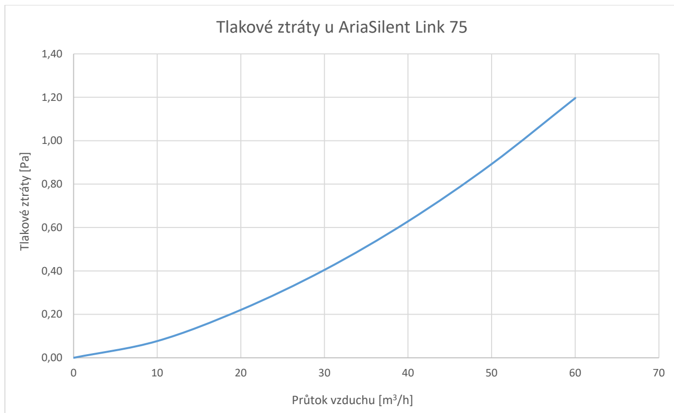
Obrázek: Tlakové ztráty u AriaSilent Link 75
