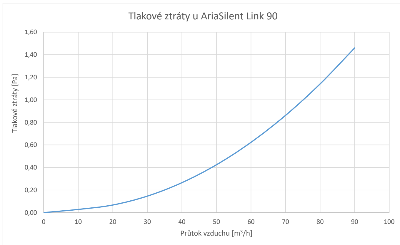
Obrázek: Tlakové ztráty u AriaSilent Link 90
