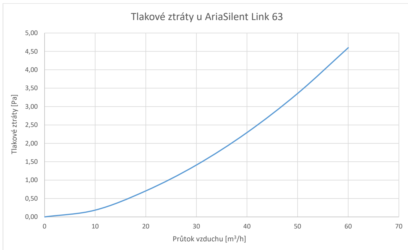
Obrázek: AriaSilent Link 63 - tlakové ztráty
