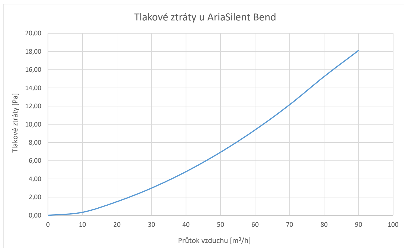
Obrázek: Tlakové ztráty u AriaSilent Link Bend
