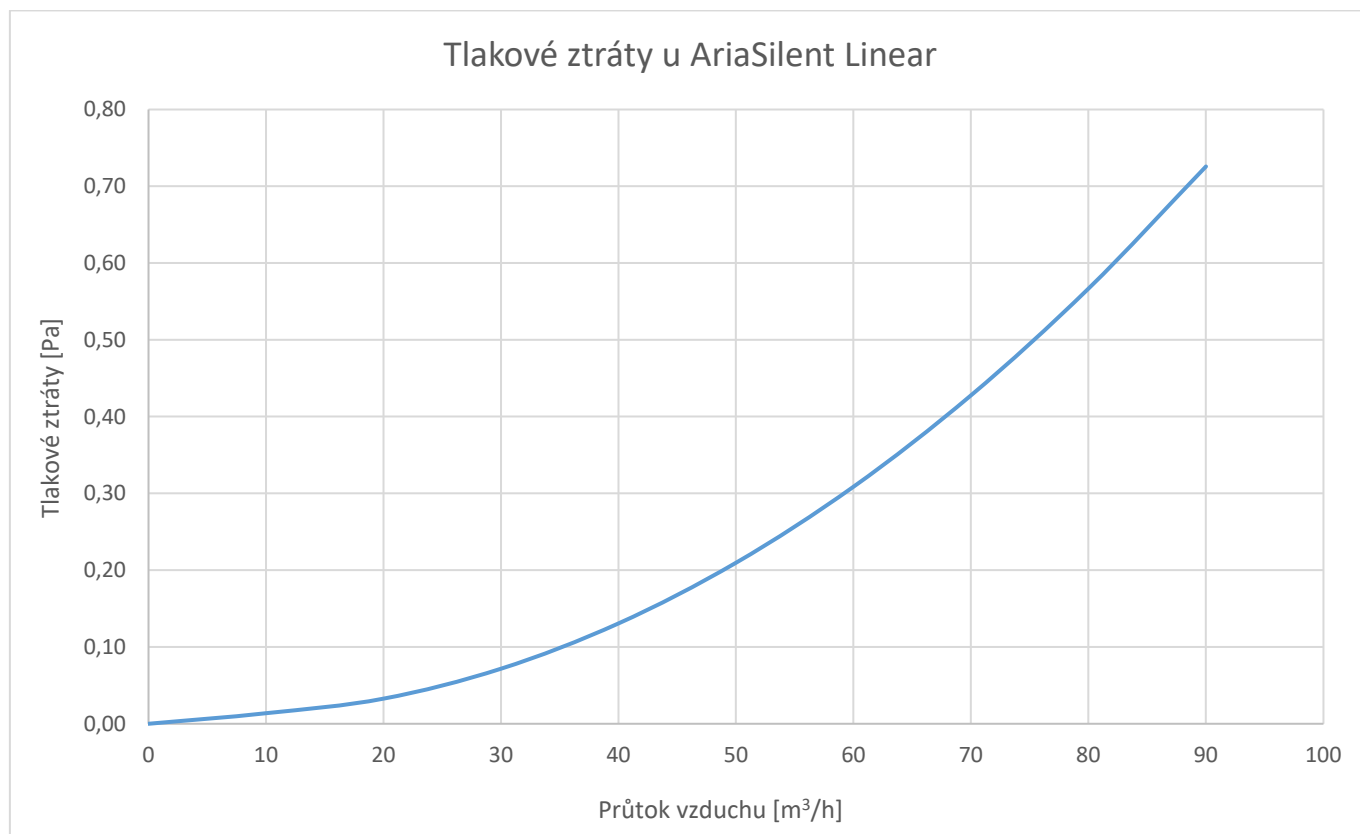
Obrázek: Tlakové ztráty u AriaSilent Link Linear
