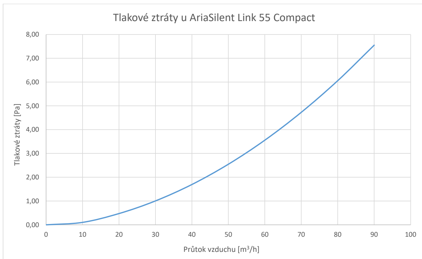
Obrázek: Tlakové ztráty u AriaSilent Link Compact 55
